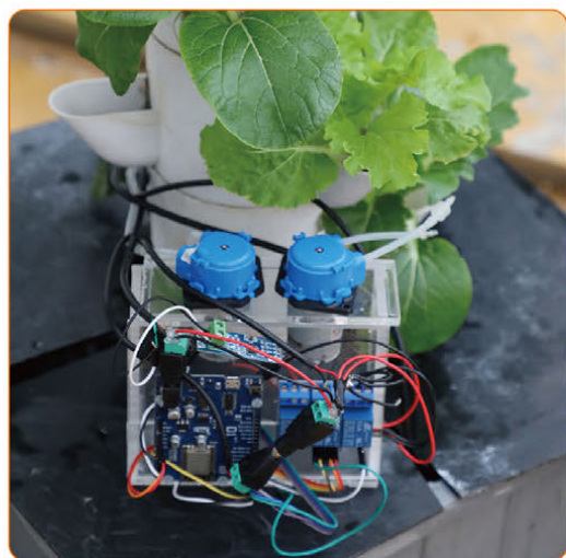
△ 運用 Arduino 結合不同傳感器實時偵測並記錄植物生長
